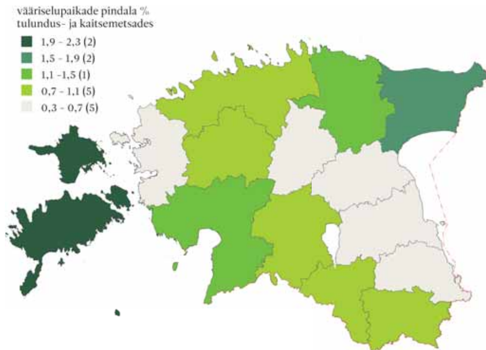
Joonis 12. Vääriselupaikade pindala suhe tulundus- ja kaitsemetsade pindalasse.
