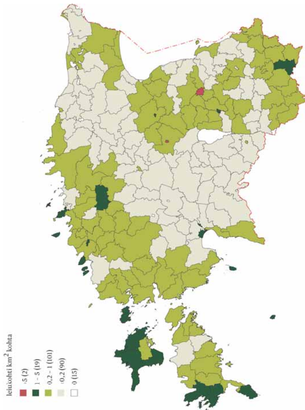
Joonis 33. Keskkonnaregistrisse kantud kaitsealuste liikide leiukohtade arv ruutkilomeetril.
