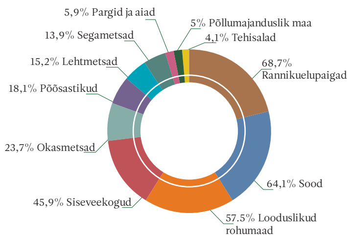
Joonis 36. Elupaikade kaitstus Eestis 2000. aasta maakatte ja 2007. aasta kaitsealuste alade seisu järgi (arvestatuna protsendina vastava elupaiga üldpindalasse).
