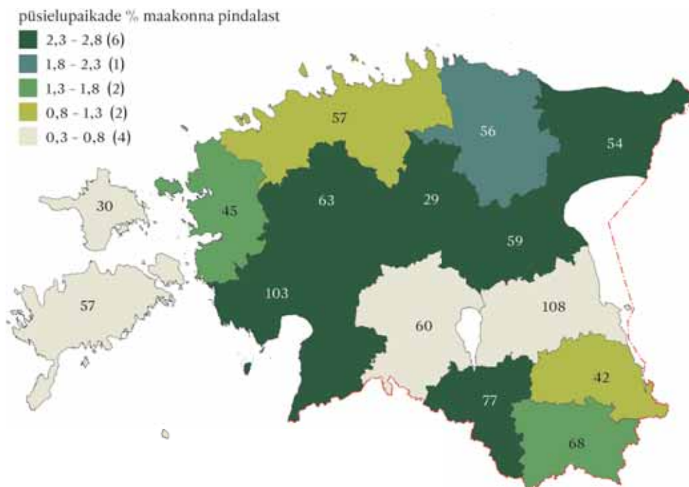
Joonis 9. Püsielupaikade osakaal maakonna pindalast. Arvestatud on vaid maismaa osa (ilma Võrtsjärve ja Peipsi järvet). Number näitab püsielupaikade arvu selles maakonnas.
