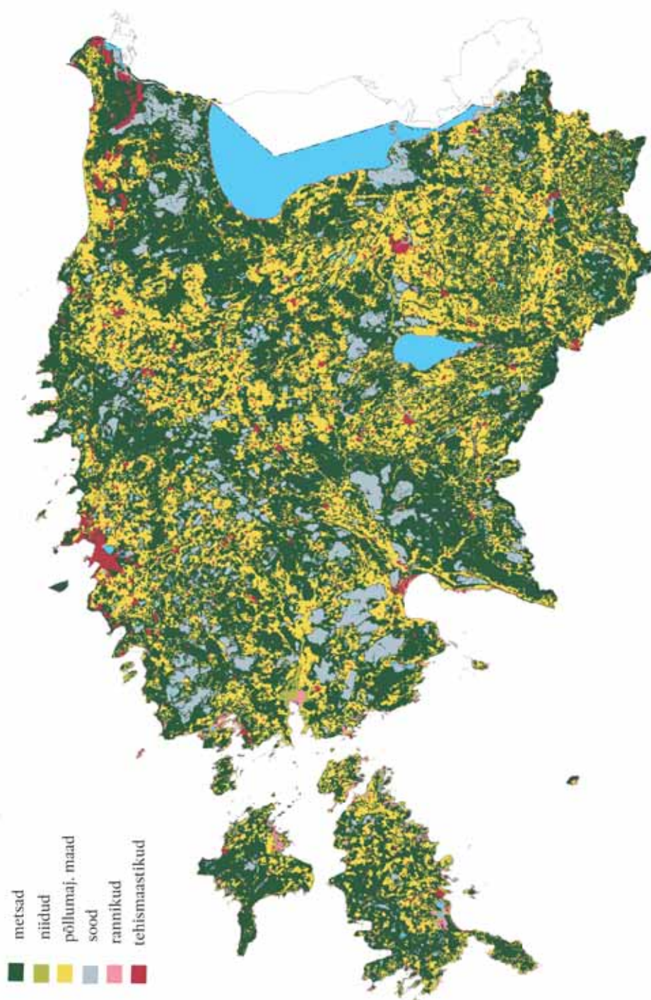
Joonis 34. Eesti maakate CORINE LandCover 2000 andmete põhjal.
