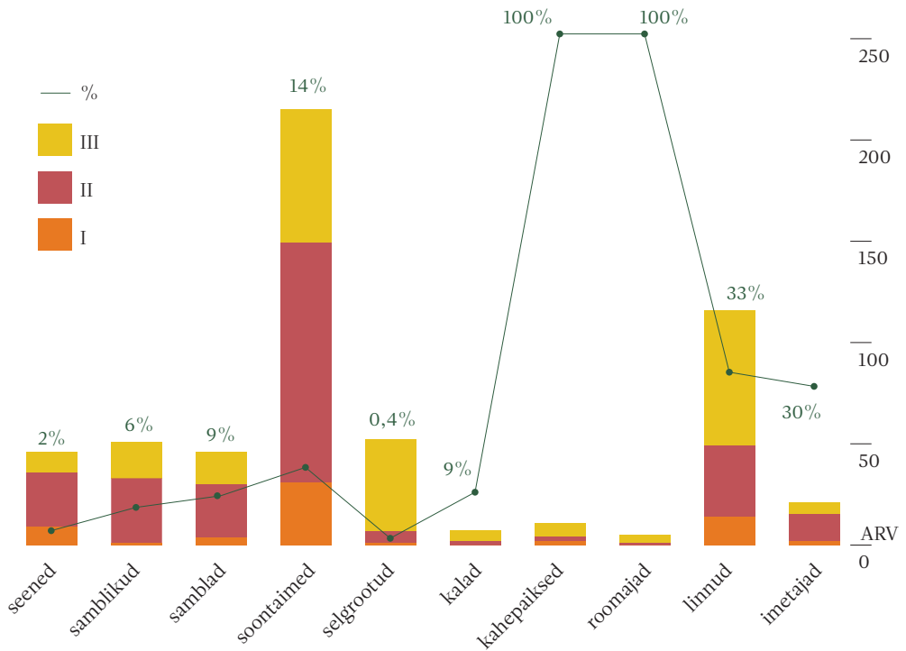
Joonis 32. Erinevatesse kaitsekategooriatesse määratud liikide arv ja nende protsent Eesti liikide koguarvust.
